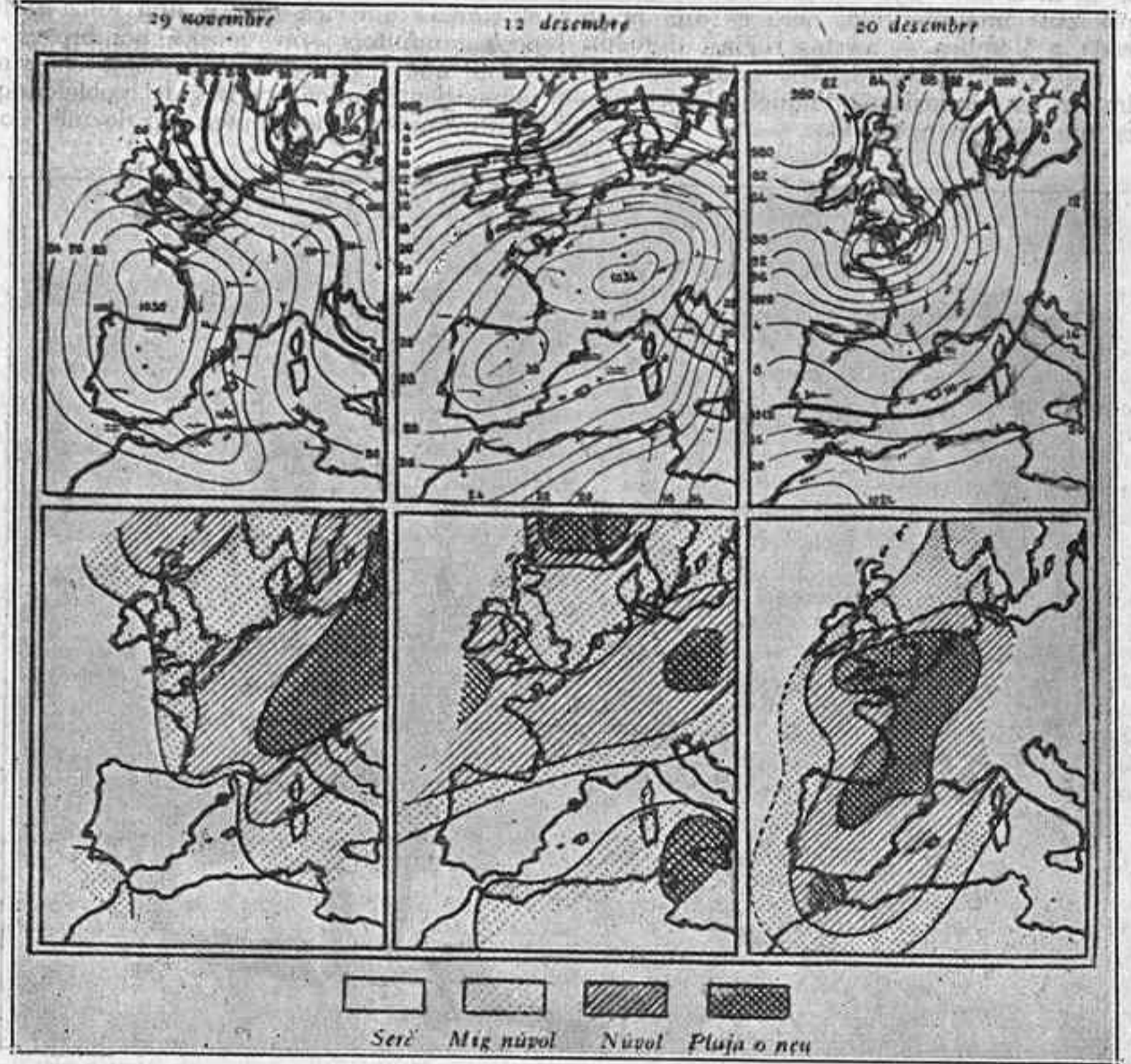
Cartes isobàriques—les de dalt—i de nulvolositat i precipitació—les de baix—del Servei Meteorològic, en les quals es veu clarament la «faixa serena» de que frueix la península (per bé que en la part central d'aquesta sovintegin les boires), que en fa la ruta aèria més afavorida atmosfèricament d'Europa.
