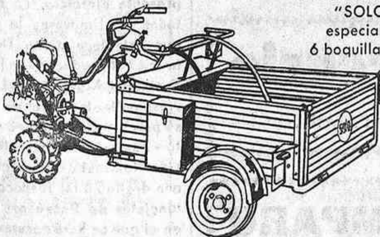
Remolque metálico adaptable a nuestra azada motorizada "SOLO" carga útil 500 Kgs.
