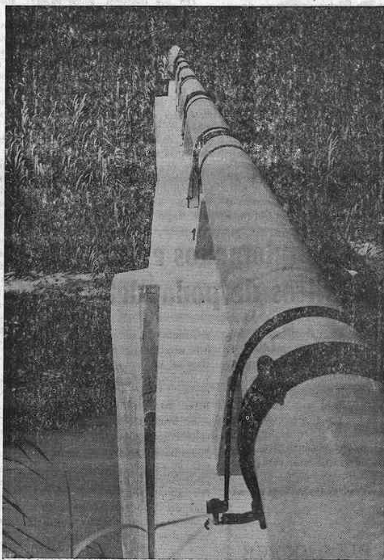
Una de las primeras conducciones de agua, construída con productos de la nueva factoría.
