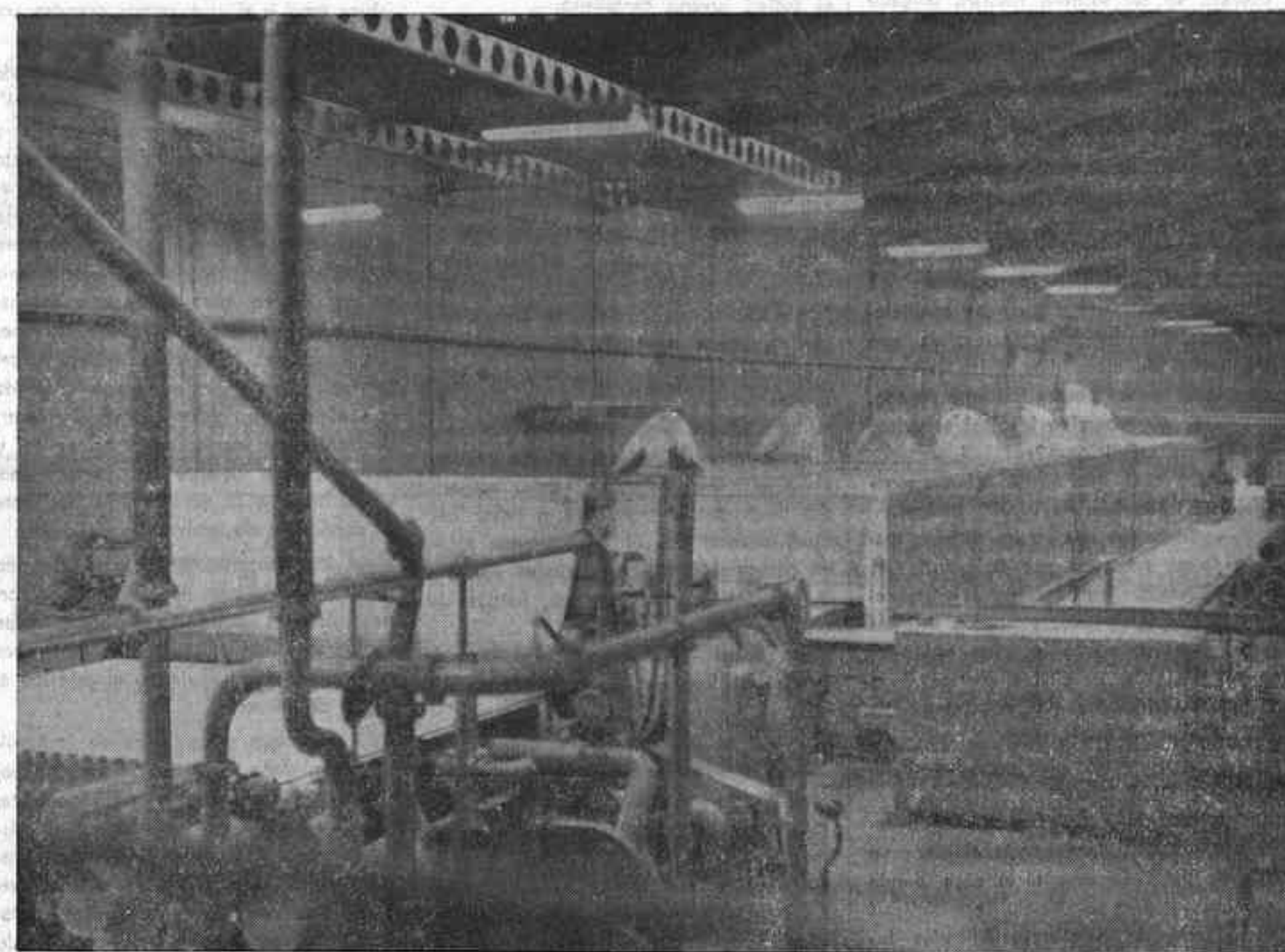
Una parte del tren de fabricación. En primer plano, la máquina constructora de tubos; en plano medio, la cámara de secado; al fondo, las piletas para la última fase del proceso de curación de productos.
