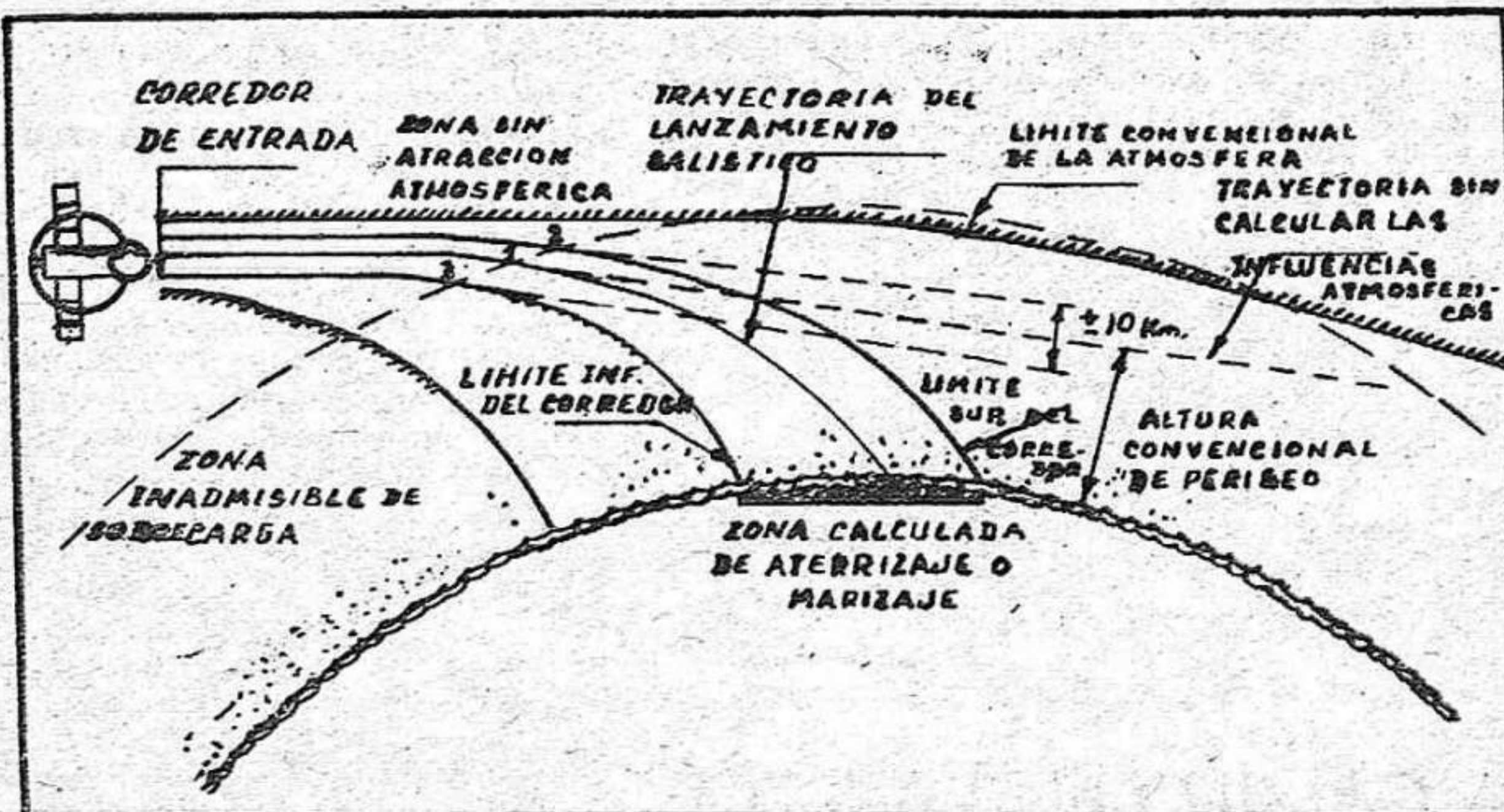
Esquema de la entrada en la atmósfera y aterrizaje. 1: Zona de entrada en la atmósfera. 2: Zona de entrada en la atmósfera con aterrizaje en el extremo de la zona calculada. 3: Zona de entrada en la atmósfera con aterrizaje en región cercana a la calculada.
