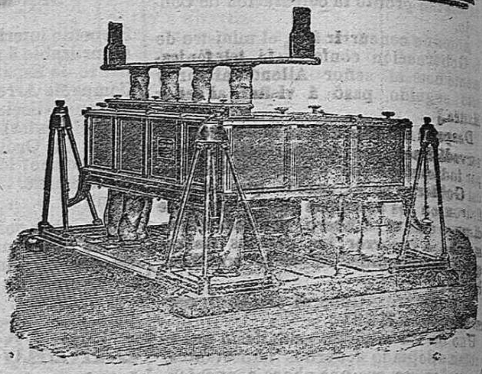
Plansichter DAVERIO construcción, 1902
