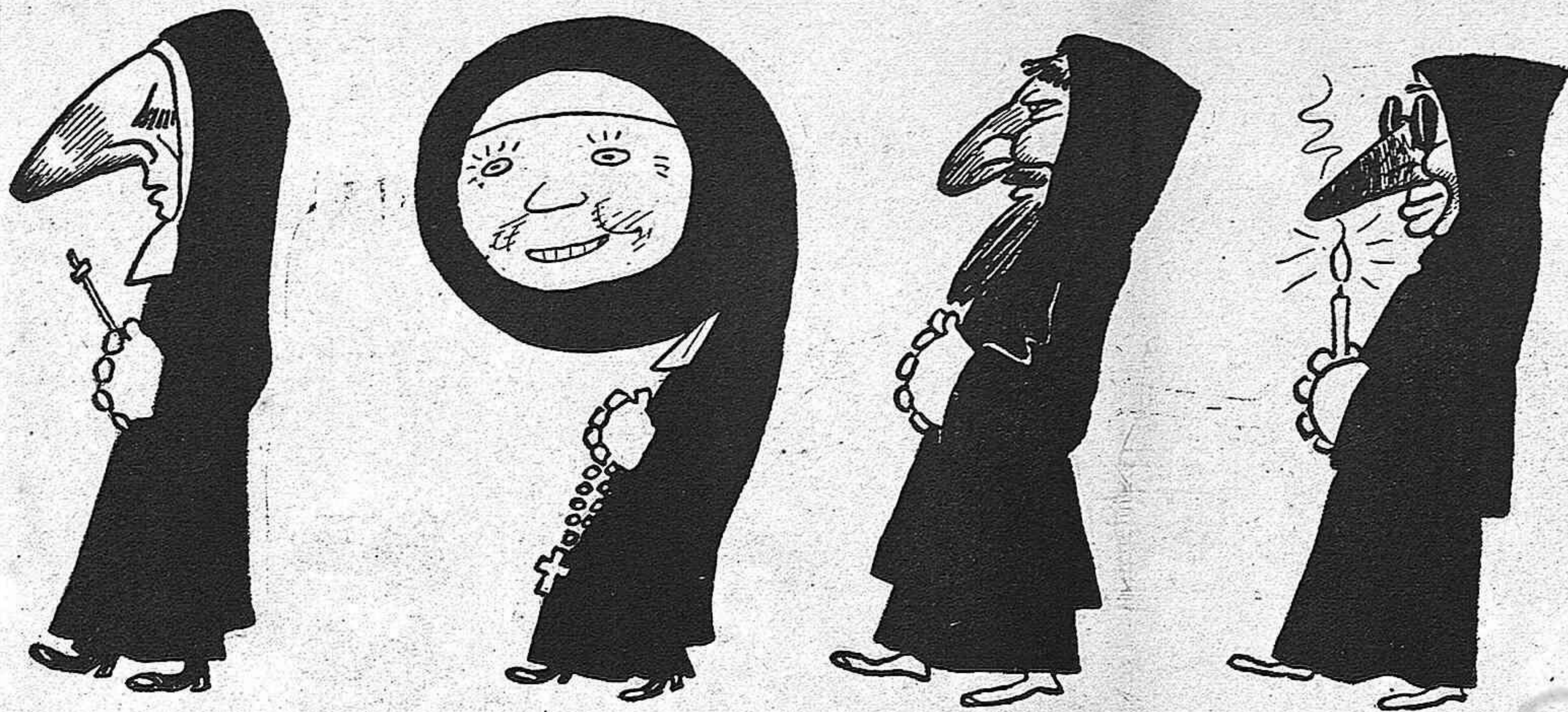
L'any espanyol.
