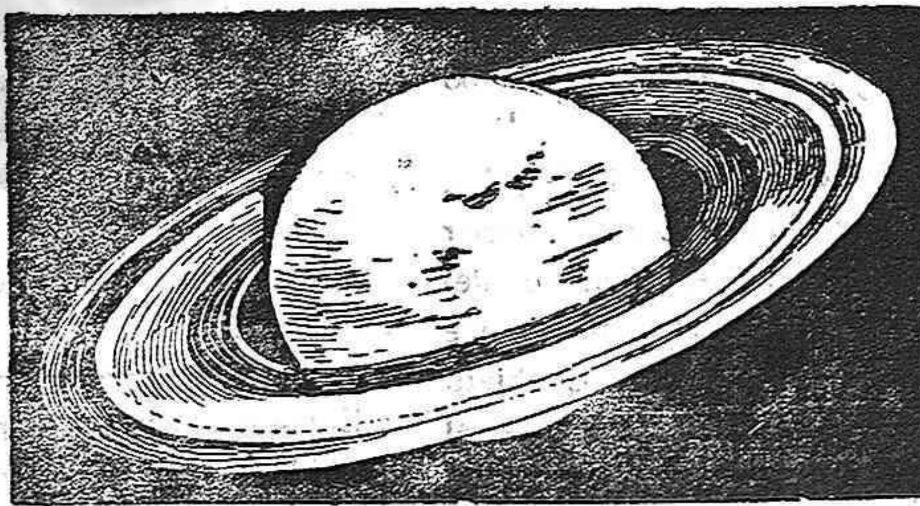
Saturno y sus anillos
