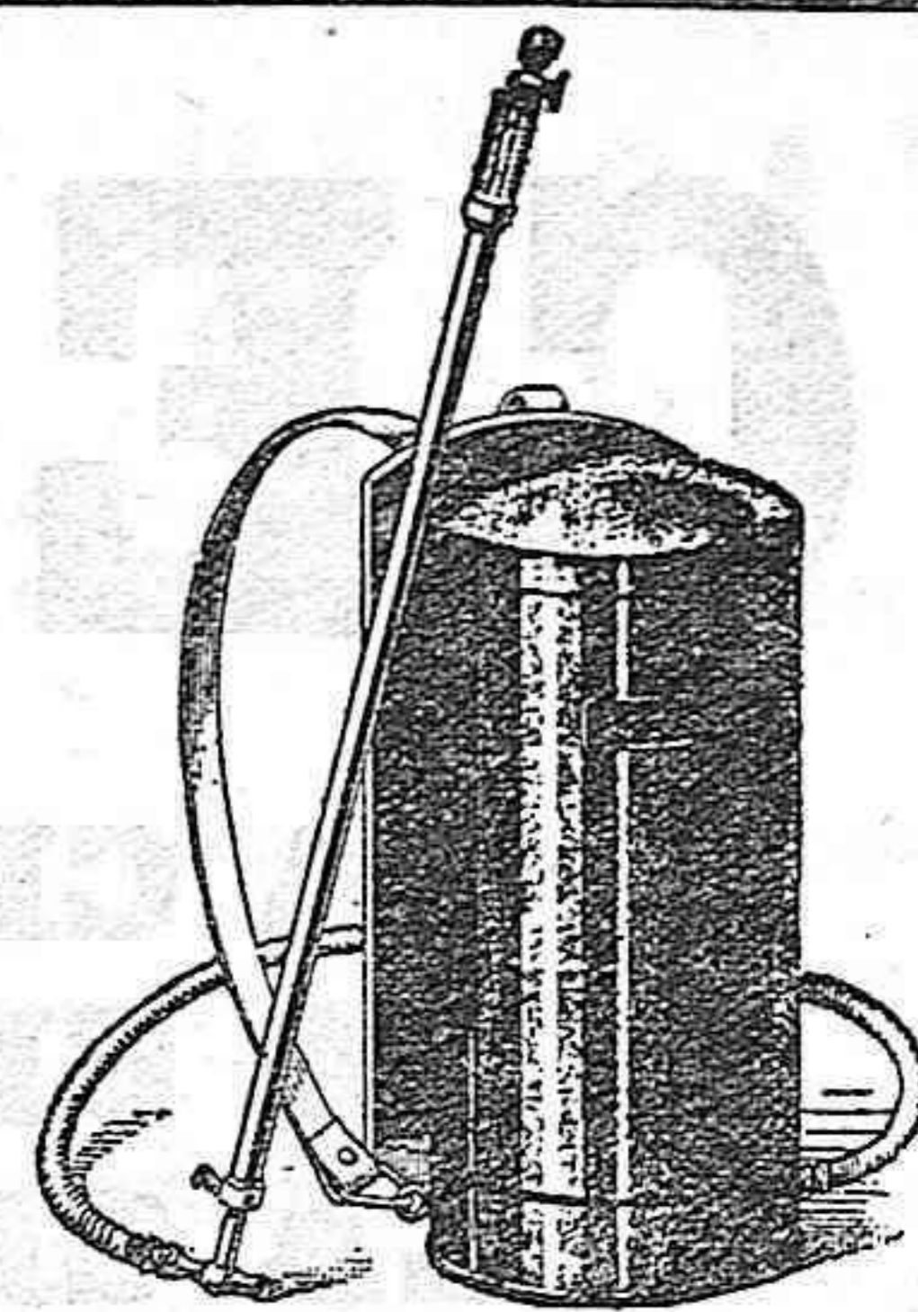
Pulverizador «LE RATIONNEL» Patentado
