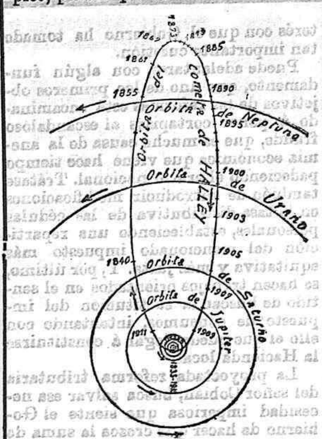
La órbita de Halley.
