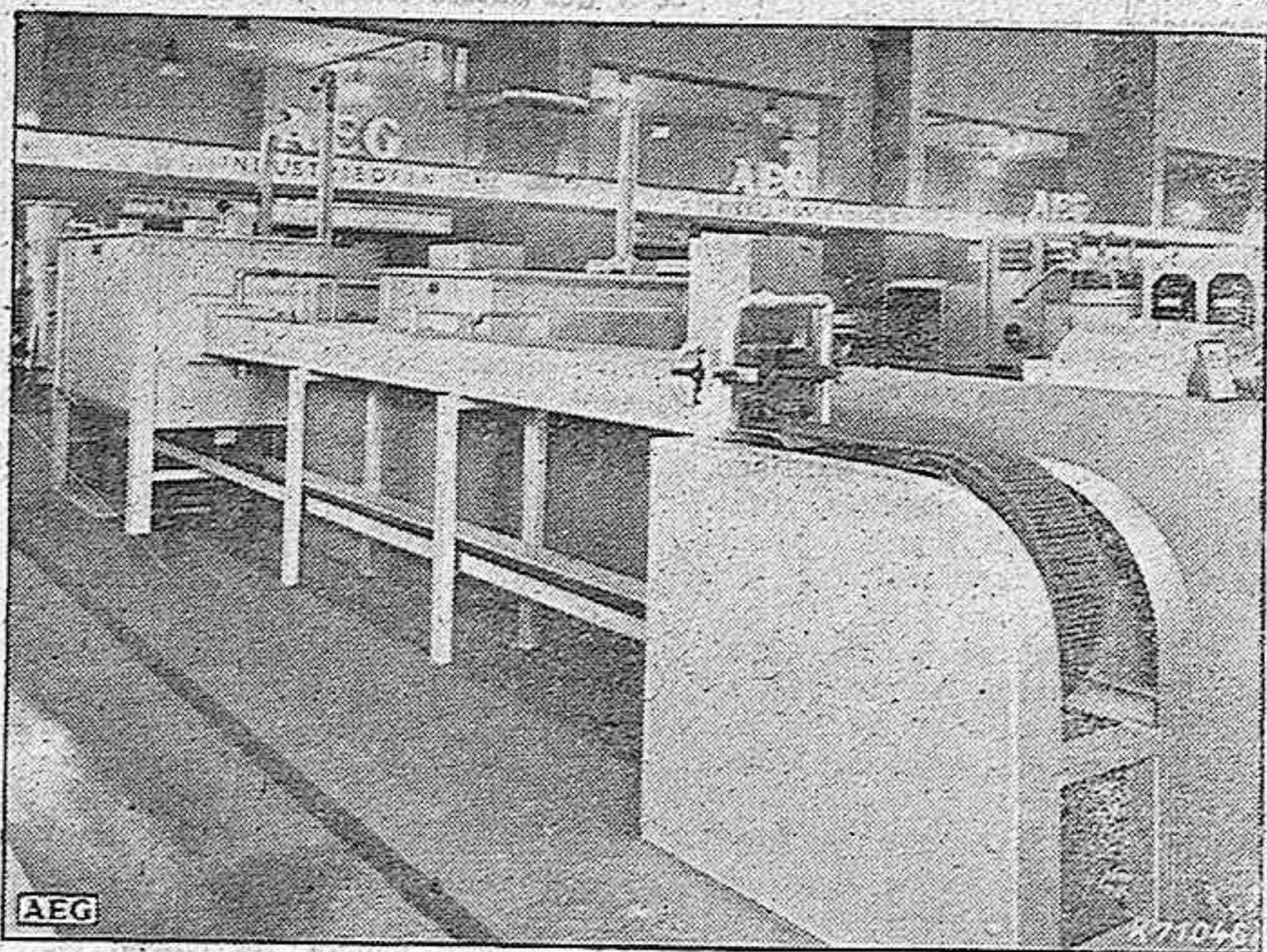
En el horno continuo con cinta de transporte, para recocer pequeñas piezas se emplea una cinta sin fin de tela metálica resistente. El retorno de la cinta se efectúa también en el interior del horno. De esta forma se logra que la cinta se enfríe poco, reduciéndose así el gasto de corriente. Para evitar que las piezas puedan caer de la cinta, ésta se construye con bordes elevados. El accionamiento de la cinta se efectúa por un motor eléctrico, montado debajo del horno y a través de un reductor regulable sin escalones, de modo que la velocidad de transportes puede ser variado en amplios límites, es decir, se la puede adaptar a la clase, forma y material de las piezas a reconocer.
