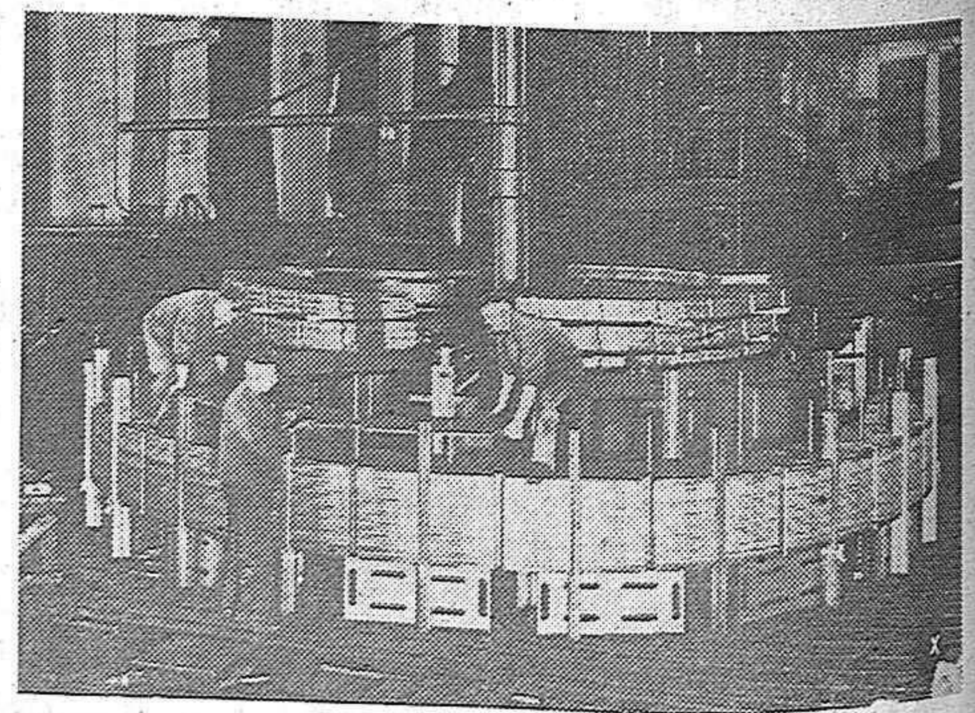
La casa A. E. G., de Alemania, acaba de construir este gigantesco generador hidráulico, de 70.000 kilovatios, para una gran Central eléctrica de Mandelbrot.
