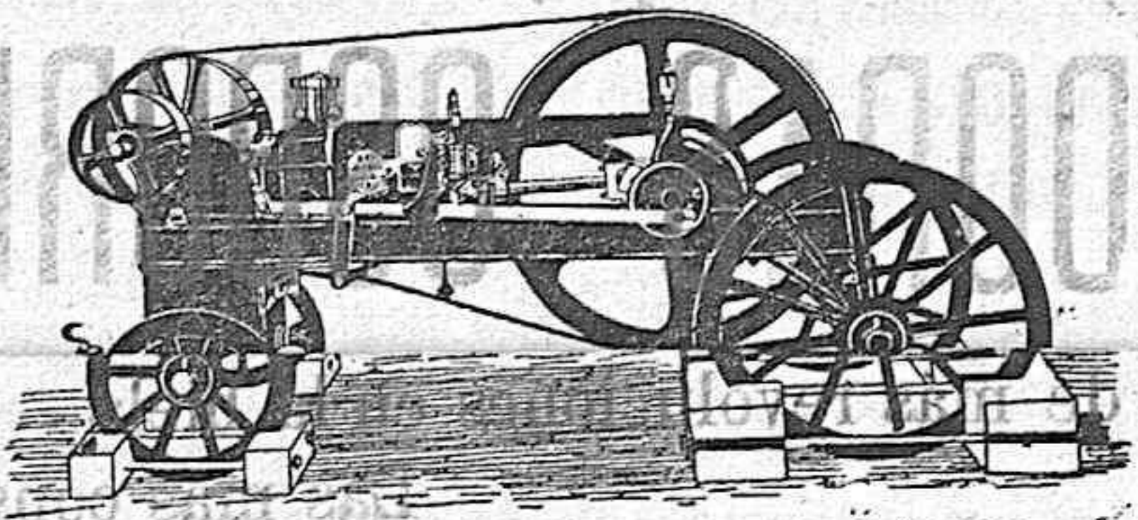
Hergomóvil de 15 H P. de fuerza para benzol
