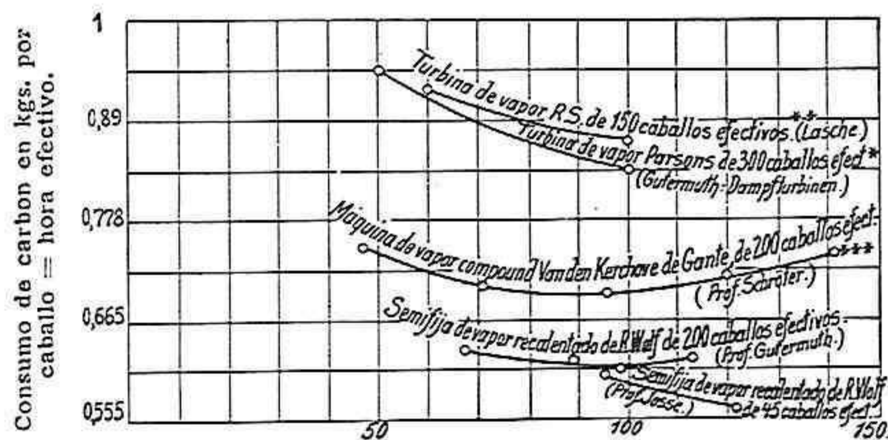
Consumo de carbon de varias máquinas de vapor á distintas cargas.
