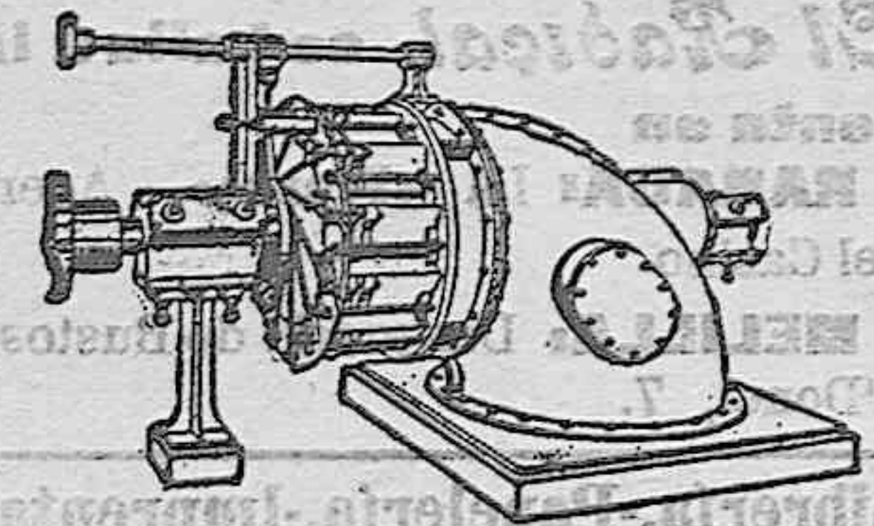
Turbina horizontal "Leffel".
