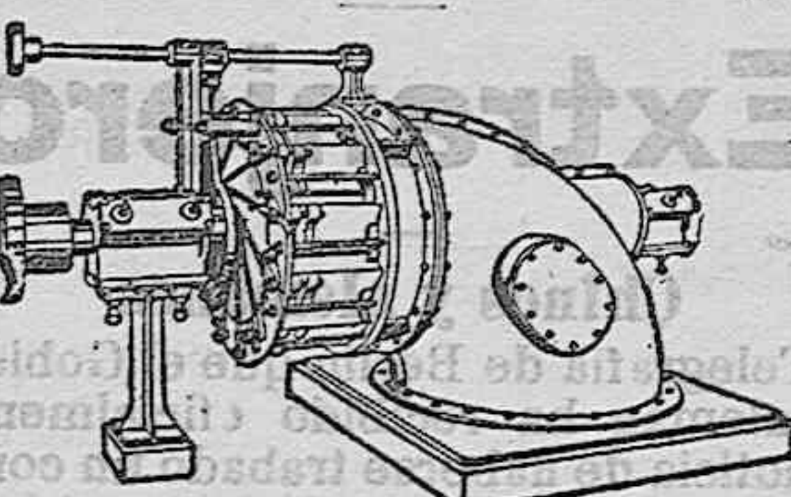
Turbina horizontal "Leffel". MOTORES DE GAS POBRE
