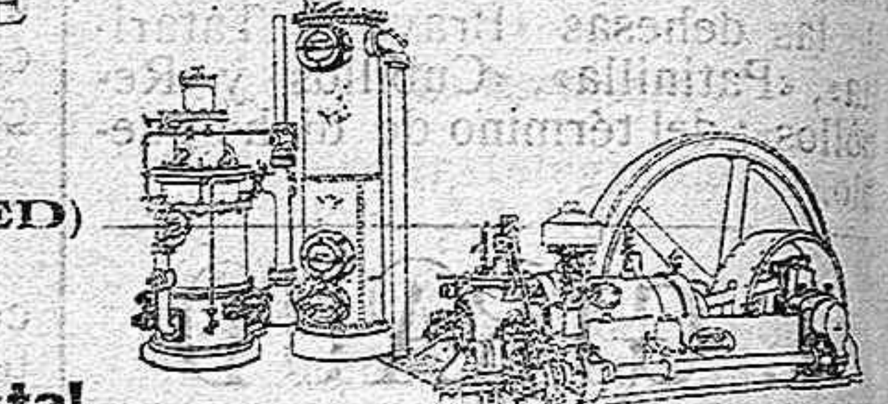
Motor de Gas Pobre por Aspiración
