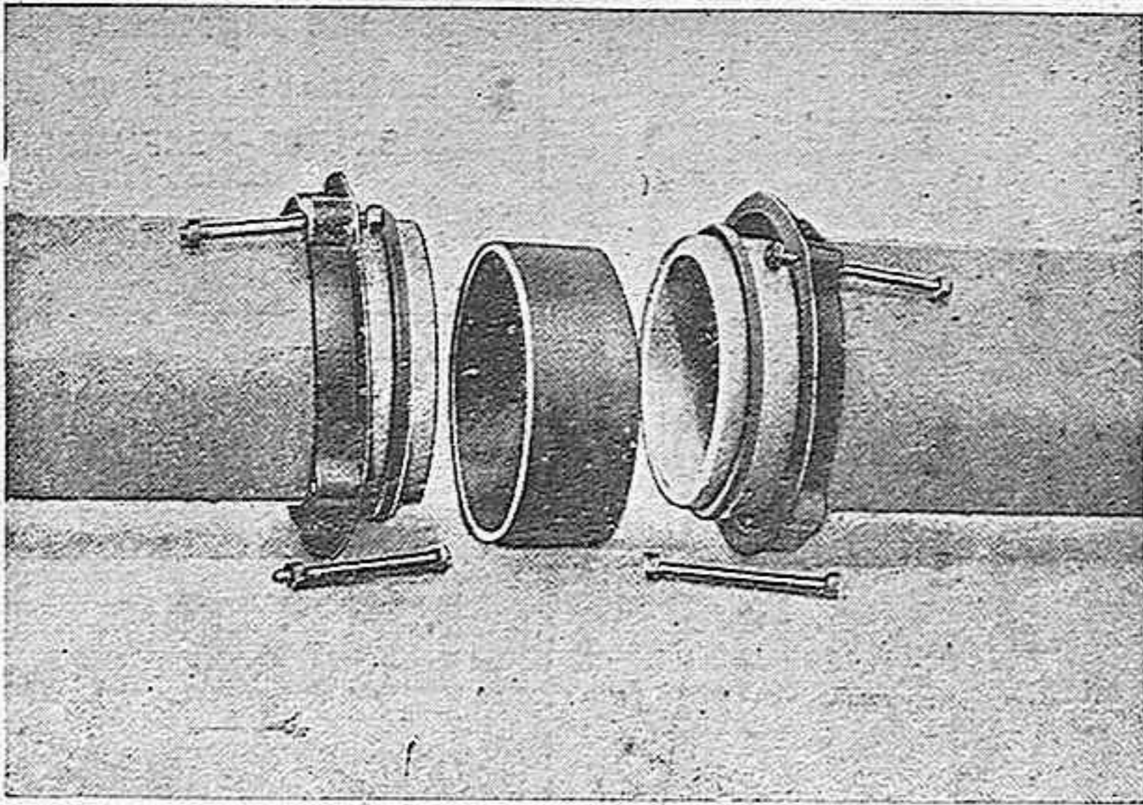
Unión sistema GIBault, desmontada.
