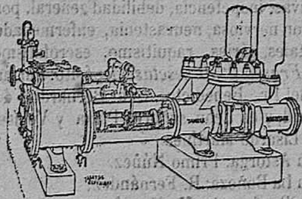
Bomba «Tangyes»
