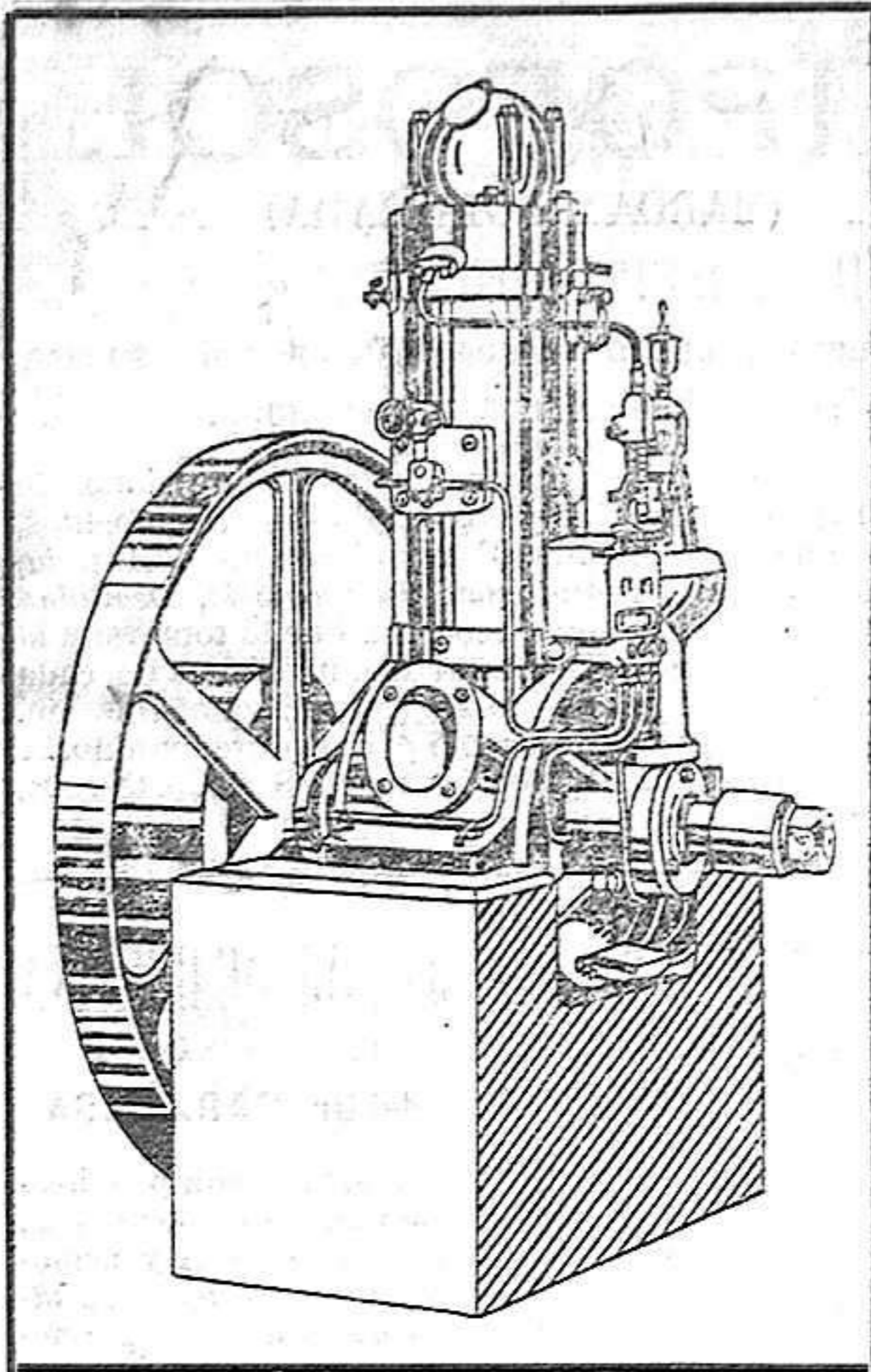
MOTOR PARA ACEITES PESADOS SIN VÁLVULAS — SIN MAGNETO
