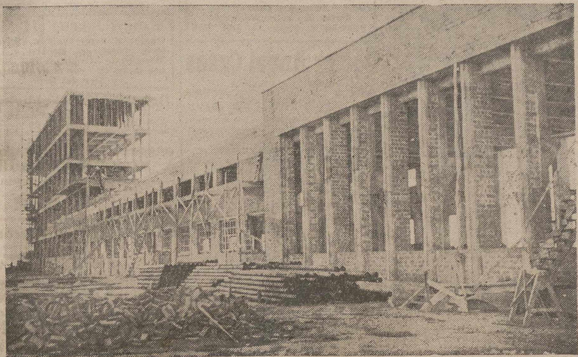
Van muy adelantadas las obras de la nueva Fábrica que se está levantando en Dueñas por la Sociedad Española de Celulosas, Fibras y Derivados, para la elaboración de papel, mediante el aprovechamiento principalmente de la paja. Se tiene la impresión de que enseguida se hará el montaje de la maquinaria, para comenzar a funcionar en los primeros meses del año próximo. La foto muestra el estado en que se encuentra la construcción. (Foto FAYA)
