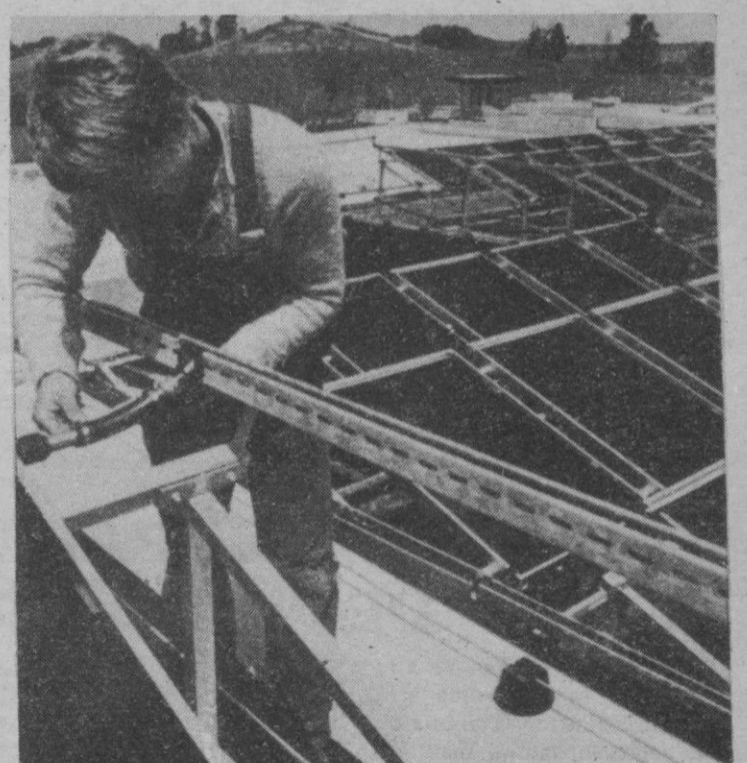
La mayor instalación de colectores solares existentes en la República Federal de Alemania acaba de ser inaugurada en la ciudad de Westfalia Ahaus y suministra calor a la gran pileta (piscina) pública de la localidad. La pileta se encuentra al aire libre y dispone de un mecanismo de oleaje artificial. En la fotografía, la instalación solar de Ahaus, que consta de 1.750 colectores. Los colectores solares aumentan, según sea la incidencia solar, la temperatura del agua en 10 grados como máximo y 5 grados como mínimo, por encima de la temperatura normal del agua. (Foto: DaDI dpa)
