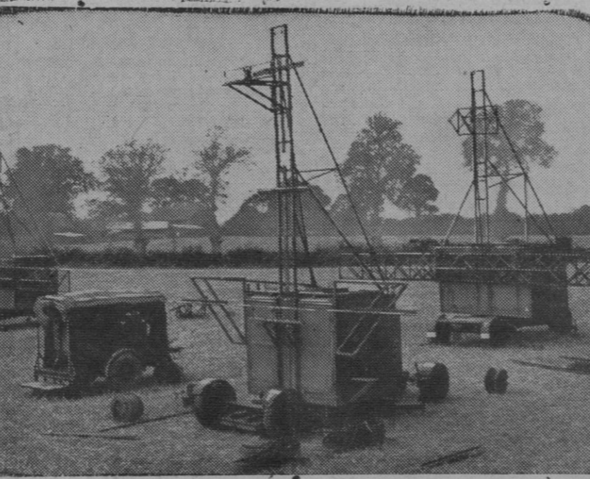
Un equipo móvil de la "Radar", perteneciente a un regimiento de artillería antiaérea (A. A.), compuesto por tres transmisores y un generador
