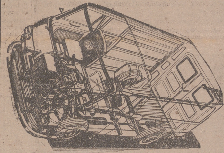
Esqueleto del nuevo modelo "COMBI-IMOSA", en el que se observa perfectamente la sincronización de los distintos elementos técnicos del motor.
