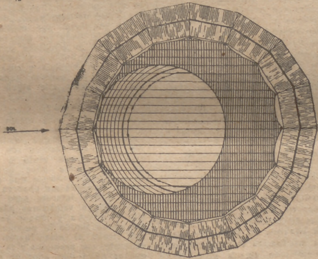
SECCION del CONJUNTO
