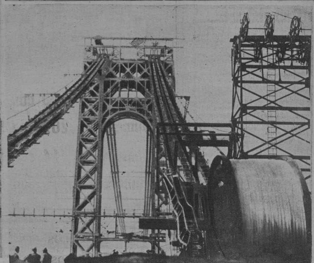
Un detalle del gran puente sobre el Hudson
