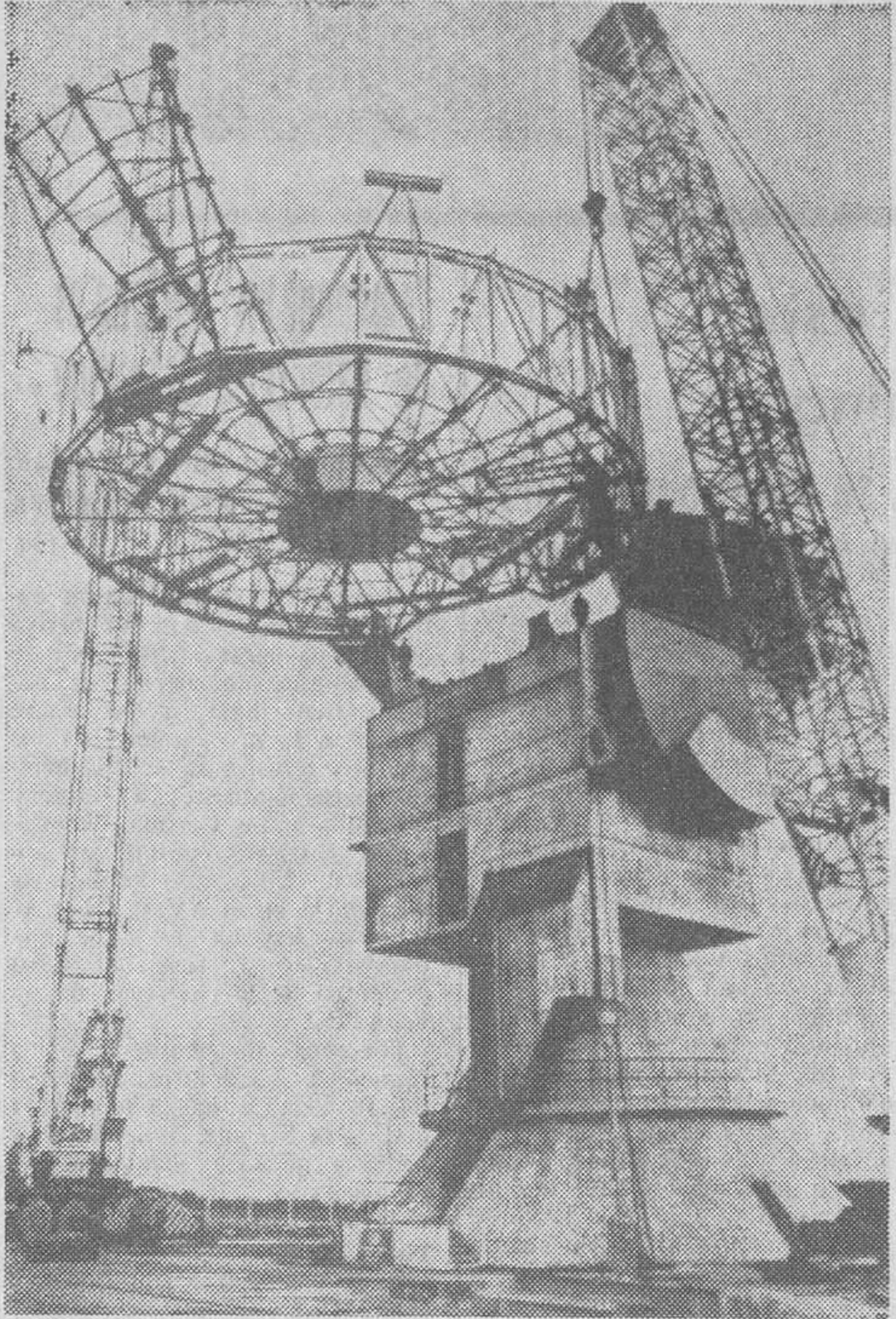
Después del famoso de Jodrell Bank, que ha recogido las primeras fotografías enviadas desde la Luna por el "Luna IX", se está construyendo ahora un nuevo radiotelescopio en Inglaterra, cuya fotografía ofrecemos a nuestros lectores, en el momento del montaje del disco de 35 toneladas de acero. — (Foto FIEL)
