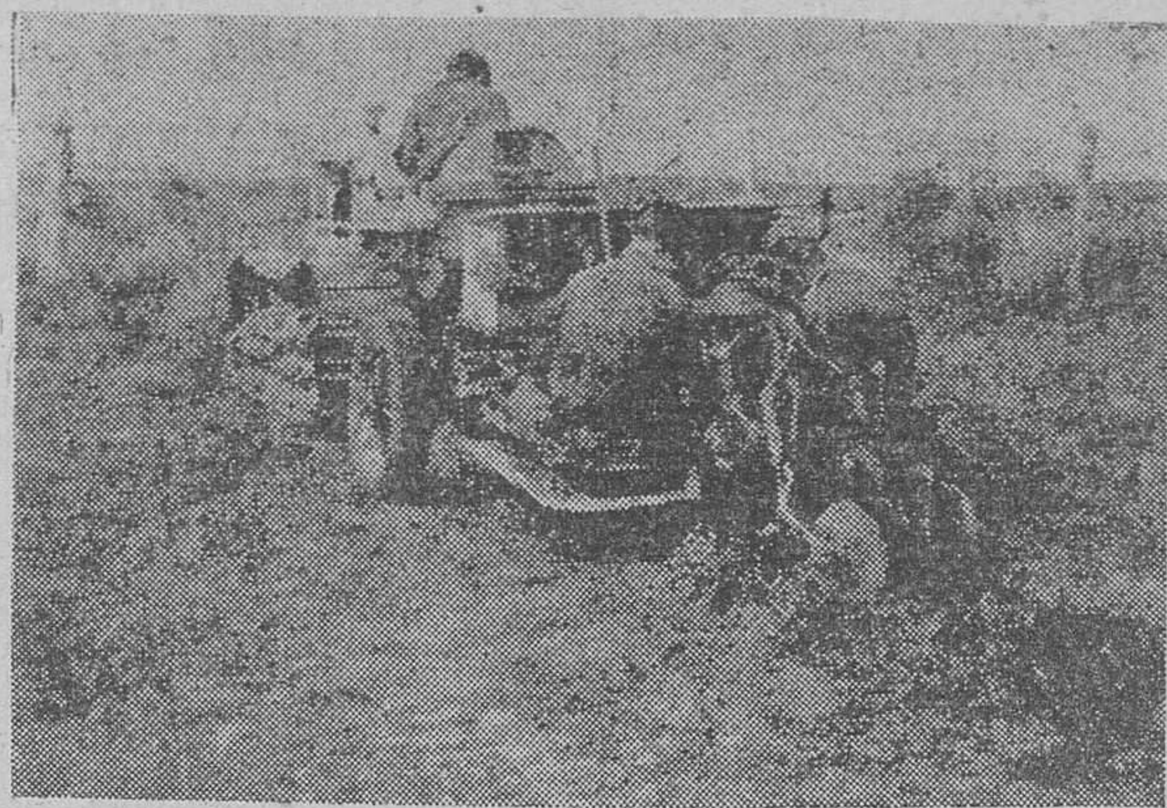
Esta máquina, remolcada por un tractor oruga, es manejada por cuatro hombres, y planta en una hora un millar de renuevos.
