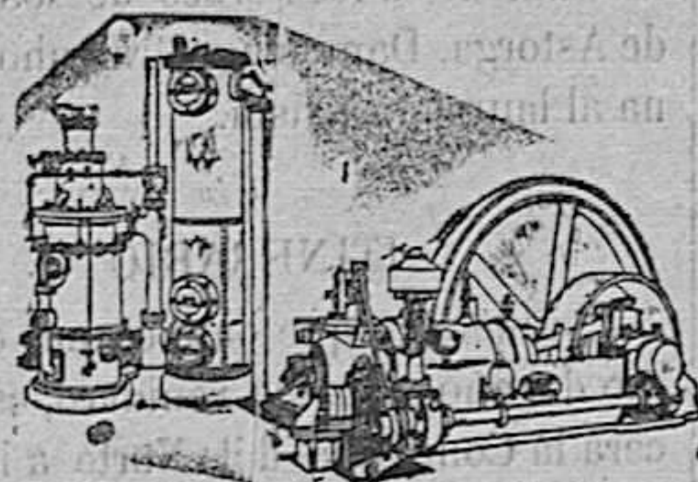
Motor de Gas Pobre por Aspiracion "Tangyes"
