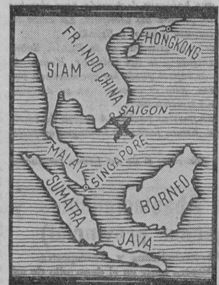
La cruz indica el lugar de la costa de Indochina, donde se ha perdido el submarino «Phenix»
