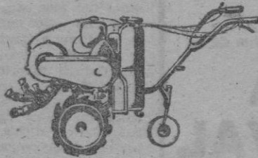
Atomizador auto-tracción «SOLO MINOR», especial para viñas 4 boquillas -5 HP. SAE
