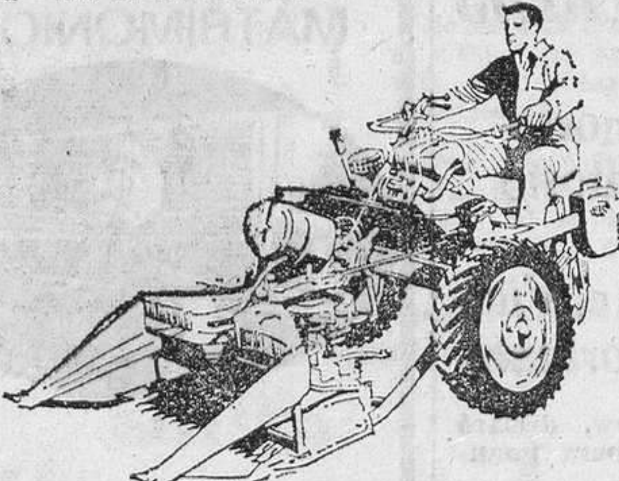
ATADORA PARA CEREAL SIN MOLINETE, PARA SITIOS CON ARBOLADO
