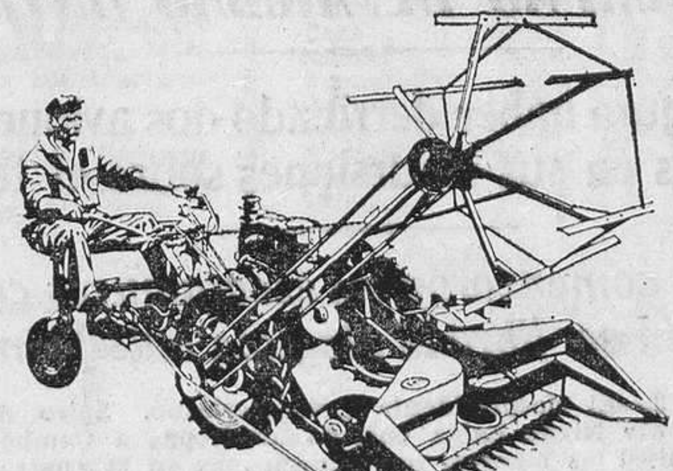
ATADORAS PARA CEREAL CON MOLINETE, PARA MIES ALTA
