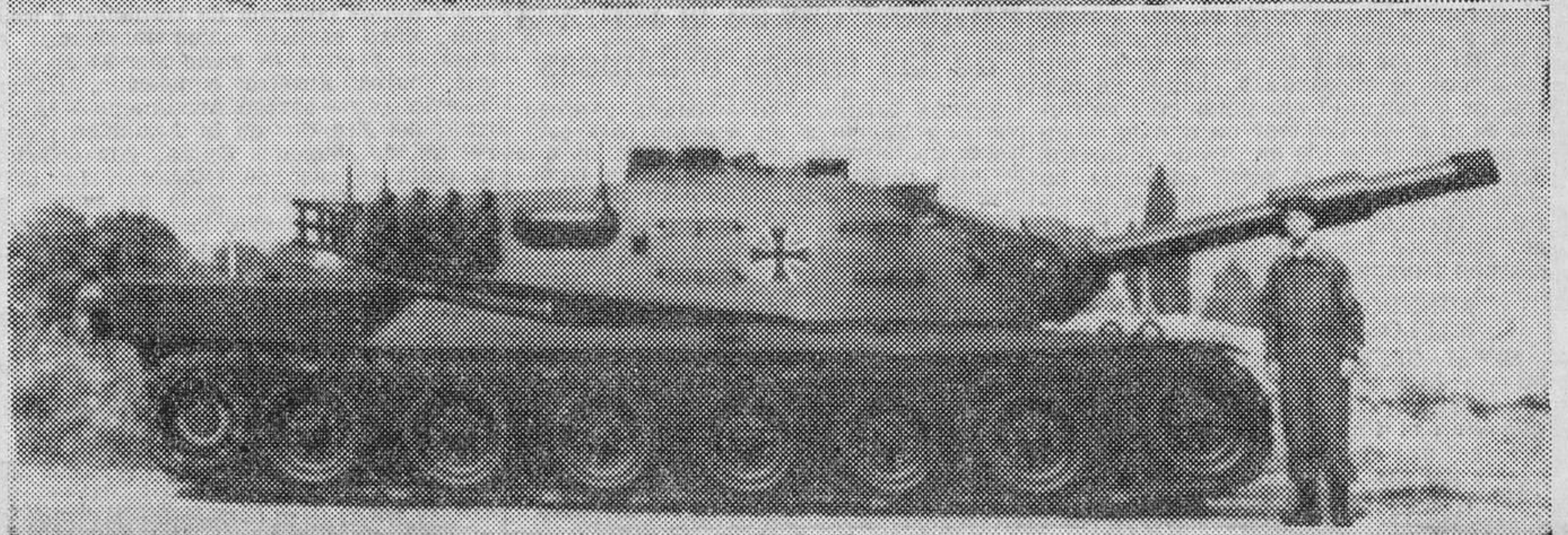
Prototipo del "Kampfpanzer 70", desarrollado conjuntamente por Estados Unidos y Alemania occidental. Se dice que es el más moderno vehículo armado del mundo occidental. El americano portacohetes del tipo "Shillelagh" y la versión alemana está equipada con un cañón totalmente automático de 120 milímetros. Tiene dos posiciones: en velocidad máxima de 75 kilómetros por hora (arriba) y en posición de lucha.
