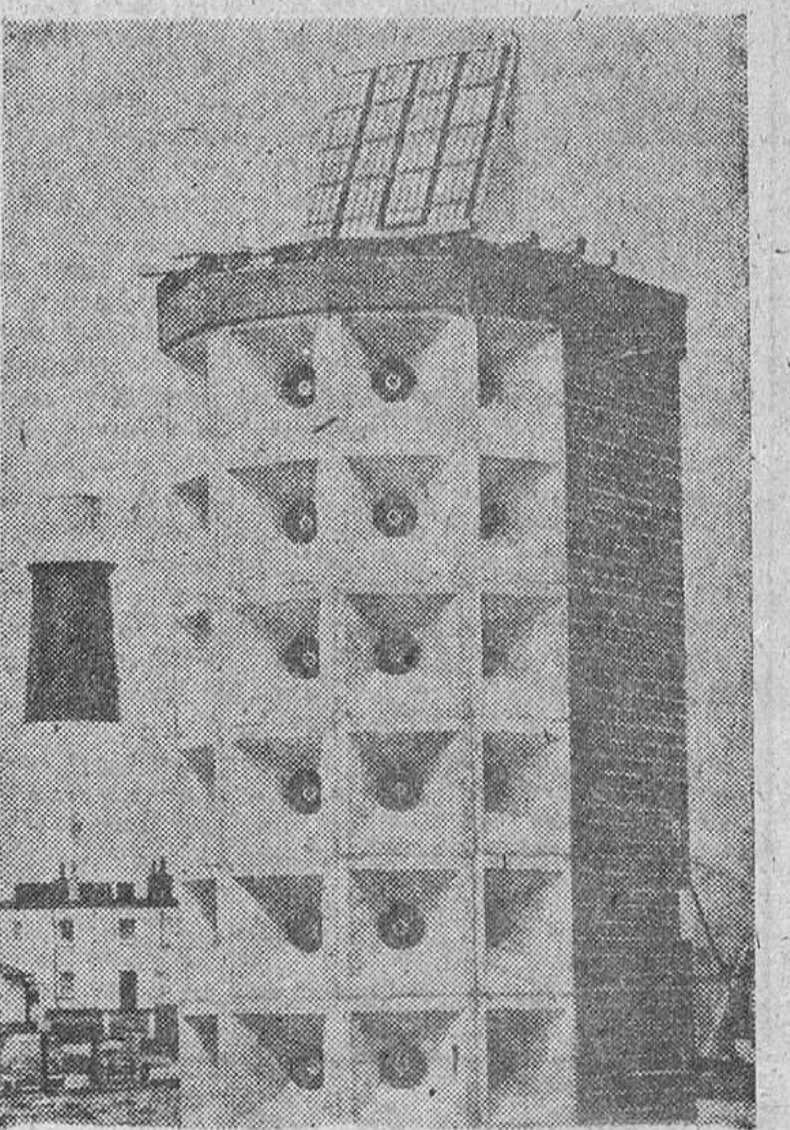
Este faro está instalado en Cornualles. Es el primero alimentado por energía solar, que proveen las baterías de los paneles encargadas de captar las radiaciones luminosas durante el día.
