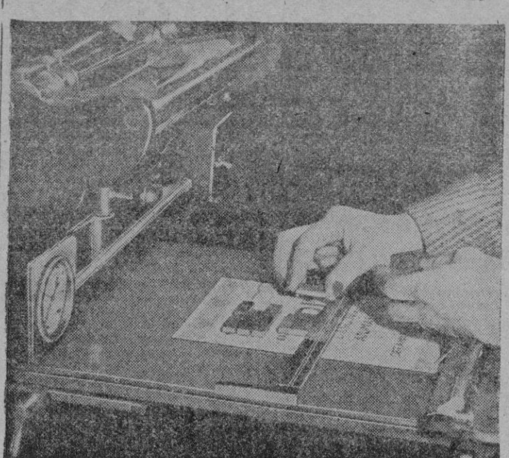
La nueva máquina para imprimir en colores, de fabricación británica, admite madera, metal, caucho, papeles de todos los gruesos, etc... y permite gran variedad de combinaciones.
