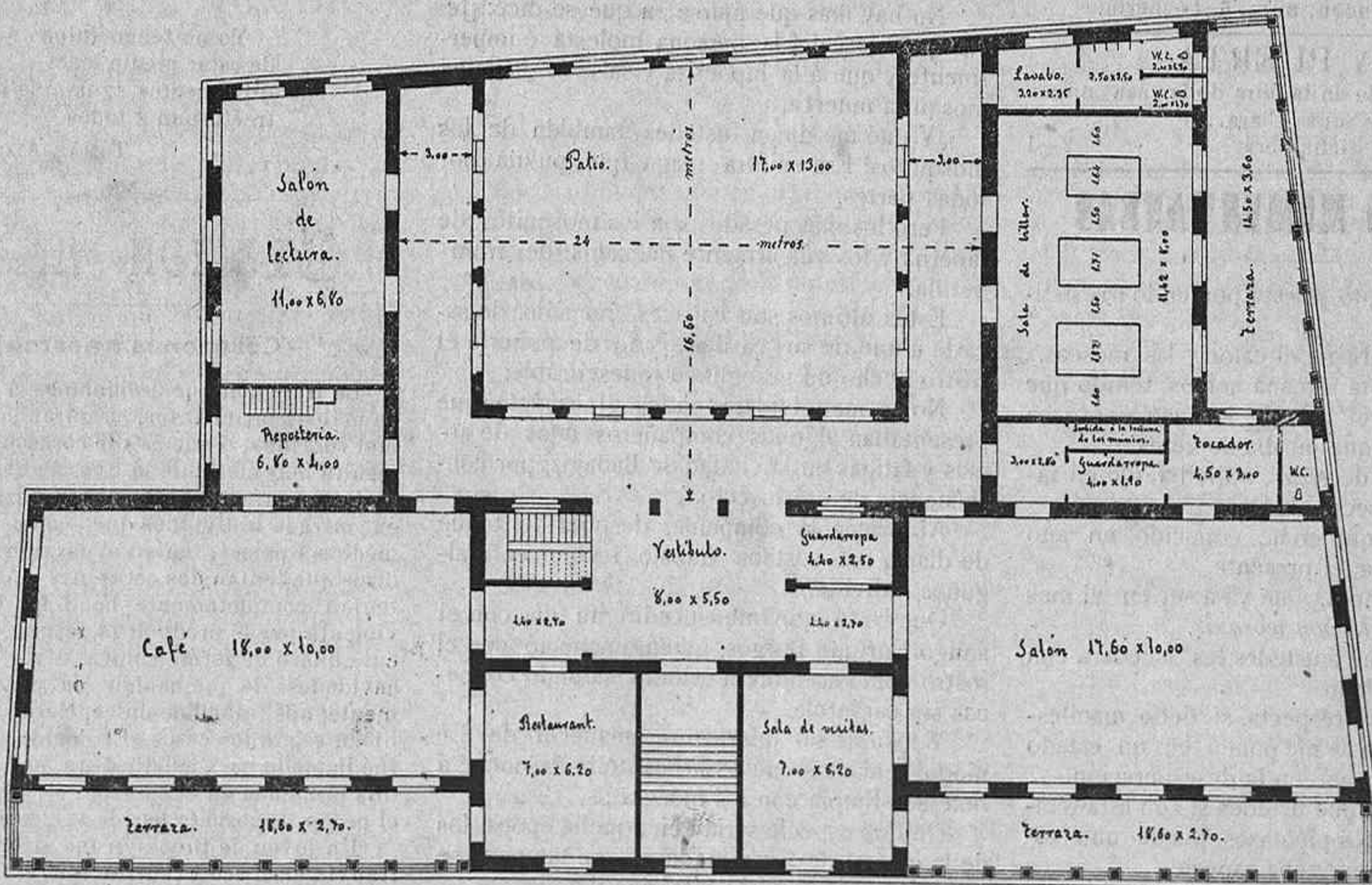
PLANTA GENERAL DEL CASINO PROYECTADO
