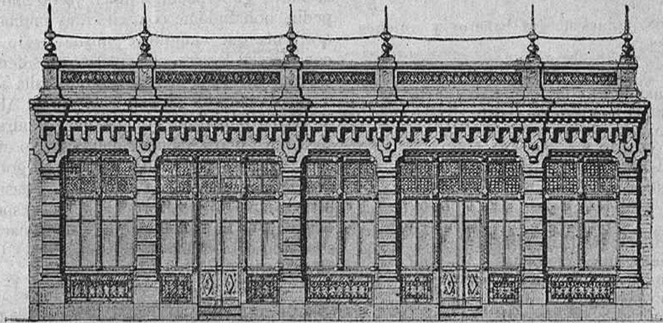
CASINO EN PROYECTO: DETALLE DE LA GALERÍA QUE CIRCUNDARÁ EL PATIO.
