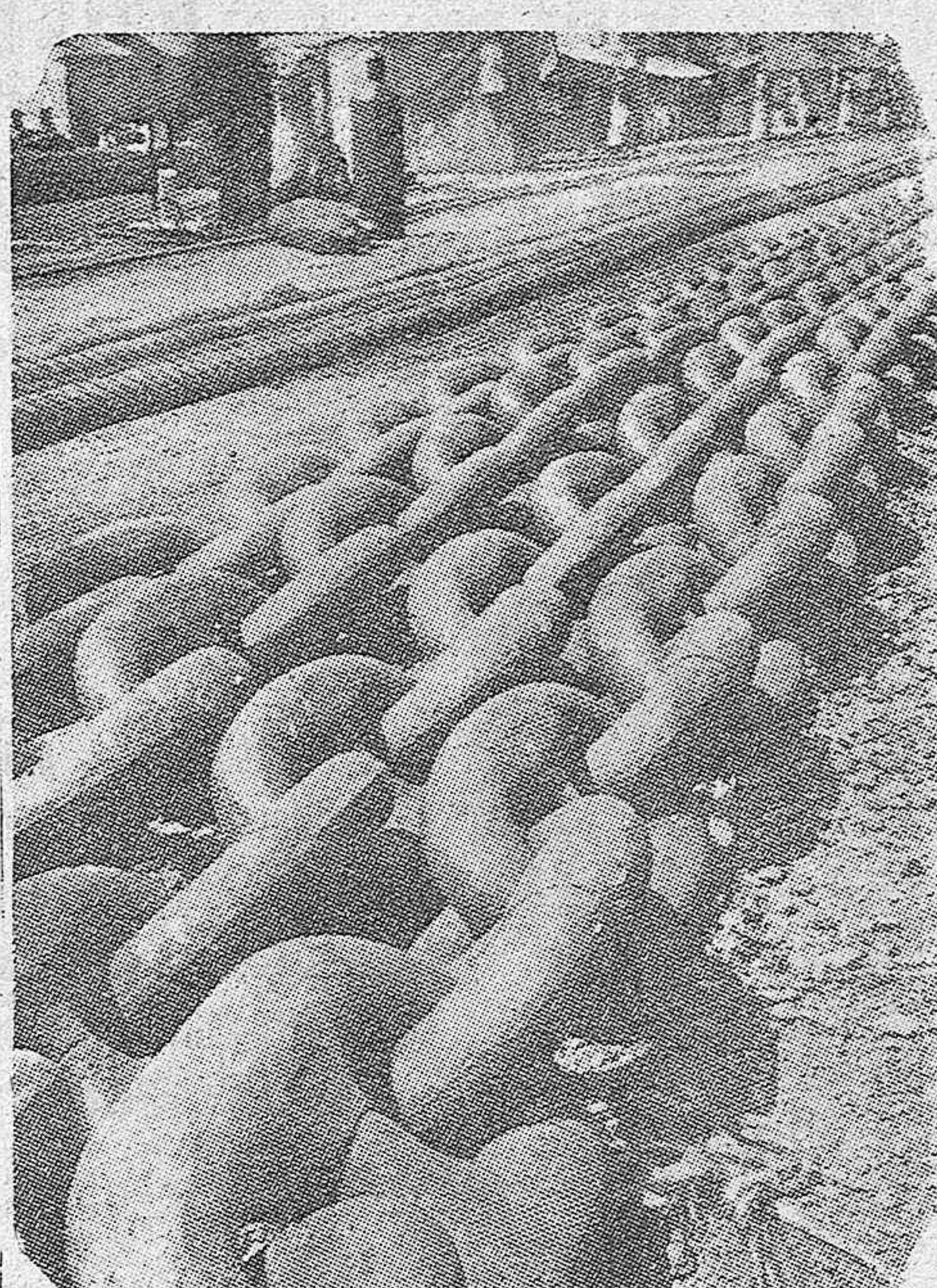
Para sacar a flote el último submarino norteamericano hundido, se utiliza un juego de cadenas, de cuya potencia da una idea la presente fotografía
