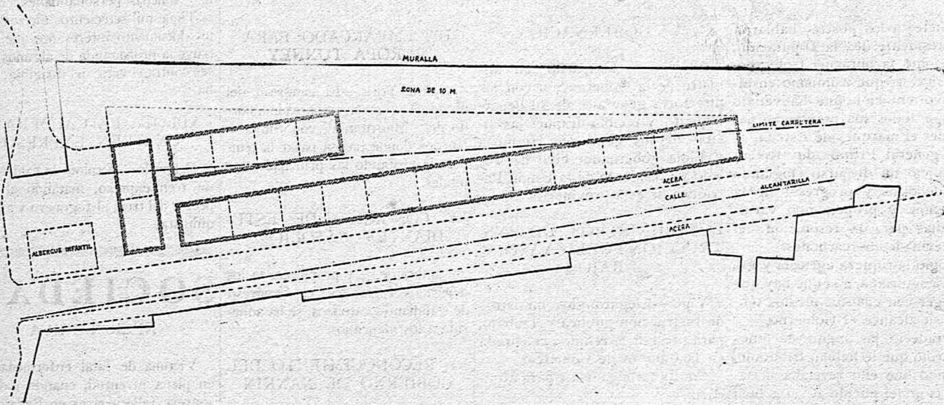
EMPLAZAMIENTO DE CASAS DE PISOS ECONOMICOS, EN LA AVENIDA DE JOAQUIN COSTA.—24 viviendas, de 114 metros cuadrados; 30, de 95 metros cuadrados. Superficie ocupada, 1.862 metros cuadrados. Importe, 465.500 pesetas.
