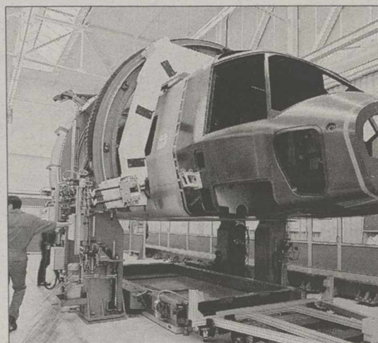
Construcción de un NH90.
