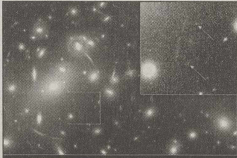
Objeto distante aumentado por la lente gravitatoria formada por el grupo de galaxias Abell 2218 (recuadro). Se trata del objeto más distante observado hasta hoy.
