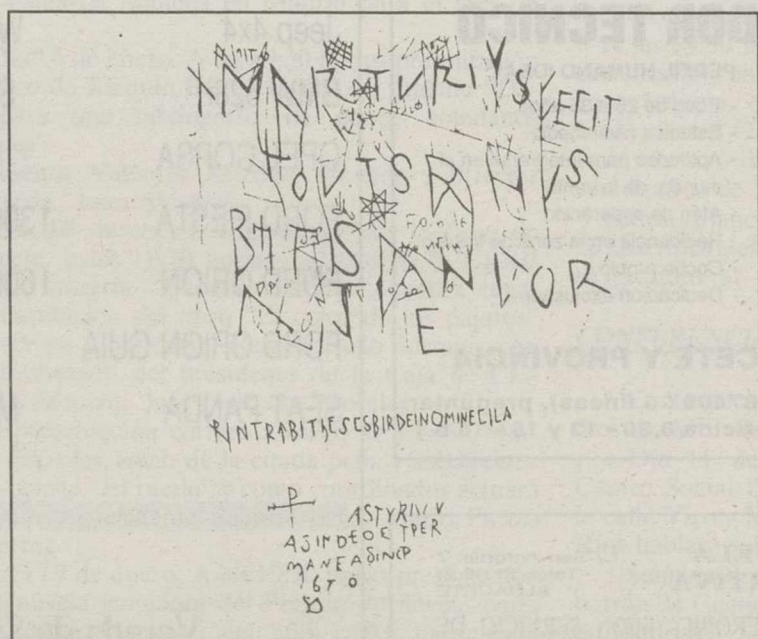
Planta, alzado e inscripciones de La Camareta, Hellín
