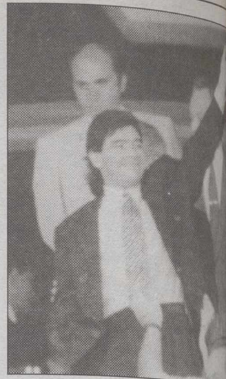
Maradona.
