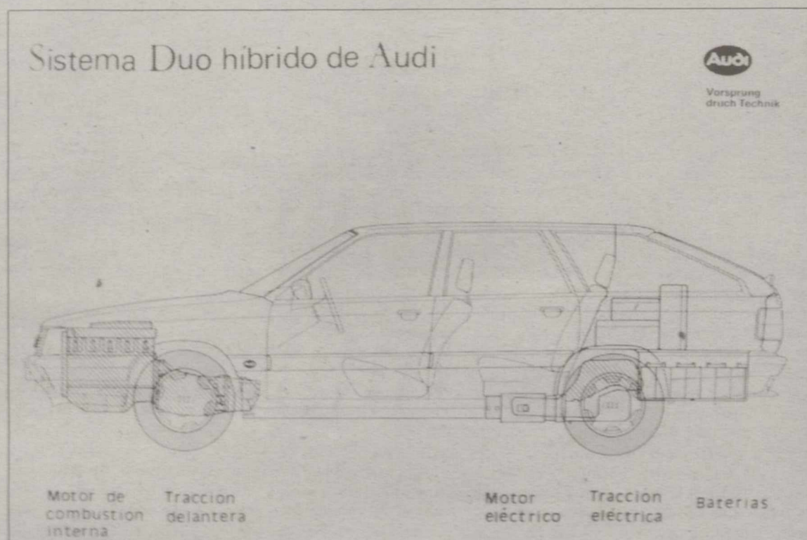
La gran novedad es que cada uno de los sistemas de propulsión actúa sobre uno de los trenes de rodaje.
