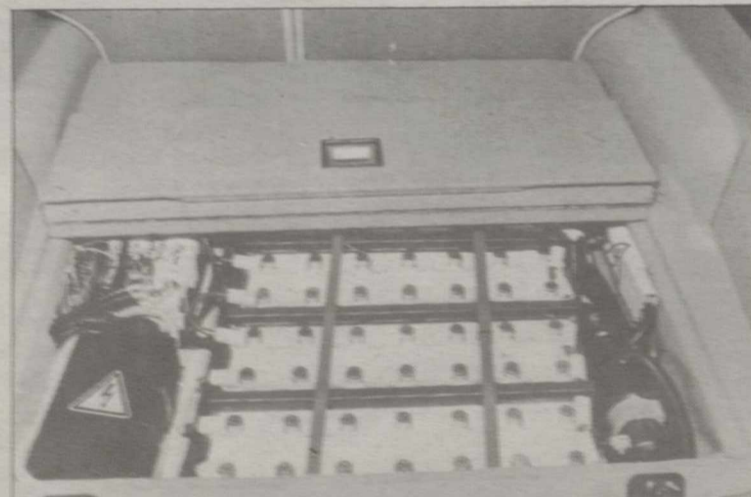
Baterías del motor eléctrico que actúa sobre el eje posterior.
