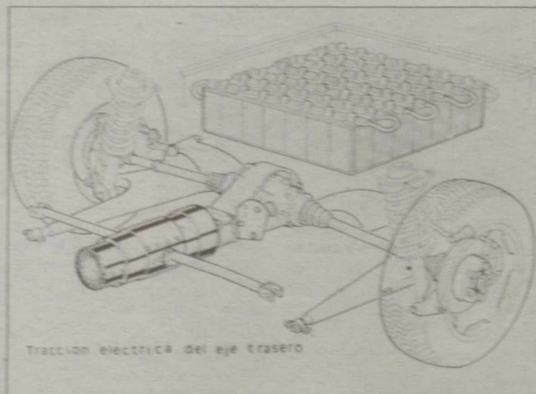
Esquema de la tracción eléctrica del eje trasero.
