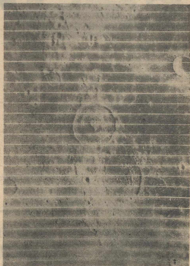
Esta foto, de resolución media, ha sido recibida en la estación espacial de Robledo de Chavela, a las 11,45 del día 19 de agosto, enviada por el vehículo espacial norteamericano «Lunar Orbiter». El área fotografiada corresponde al borde oriental de la Luna, aproximadamente a 90 grados de longitud Este y 0 grados de latitud. Esta parte de la Luna nunca había sido vista bajo el ángulo en que ha sido fotografiada esta vez. Aparecen numerosos cráteres, siendo el diámetro del gran cráter central de alrededor de 30 kilómetros. En la parte inferior izquierda aparece uno más pequeño y profundo de un diámetro de 13 kilómetros. La foto se compone de bandas de película de 35 milímetros que fueron adecuadamente dispuestas para formar el conjunto del área mostrada. (FOTO FIEL)
