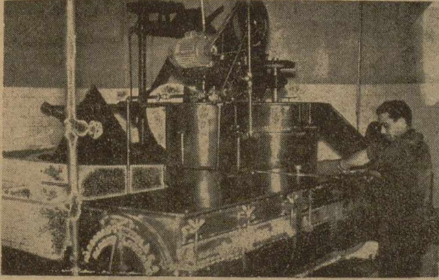
Equipo expulsor "Marzola", especial patentado.
