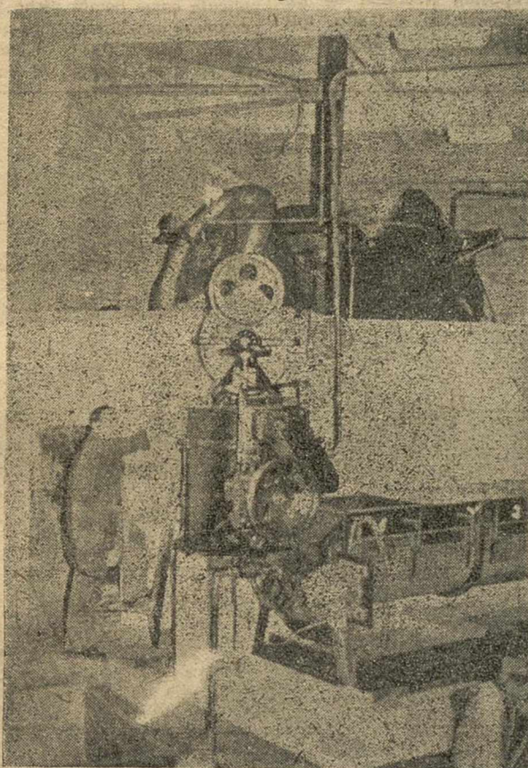
Vista de un empiedre con parte del equipo expulsor «Marzola»
