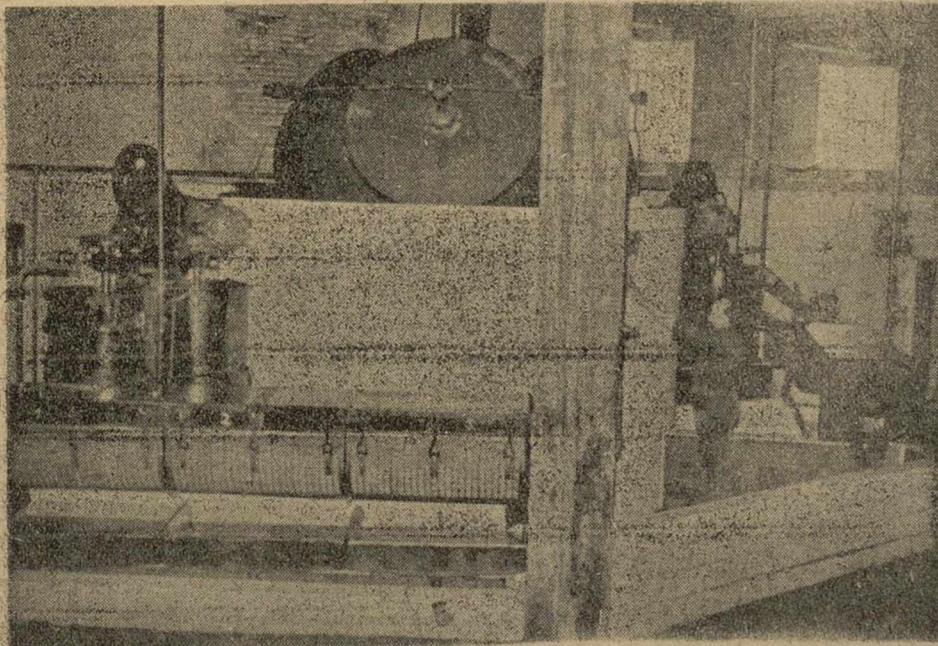
Otra vista del equipo expulsor «Marzola»
