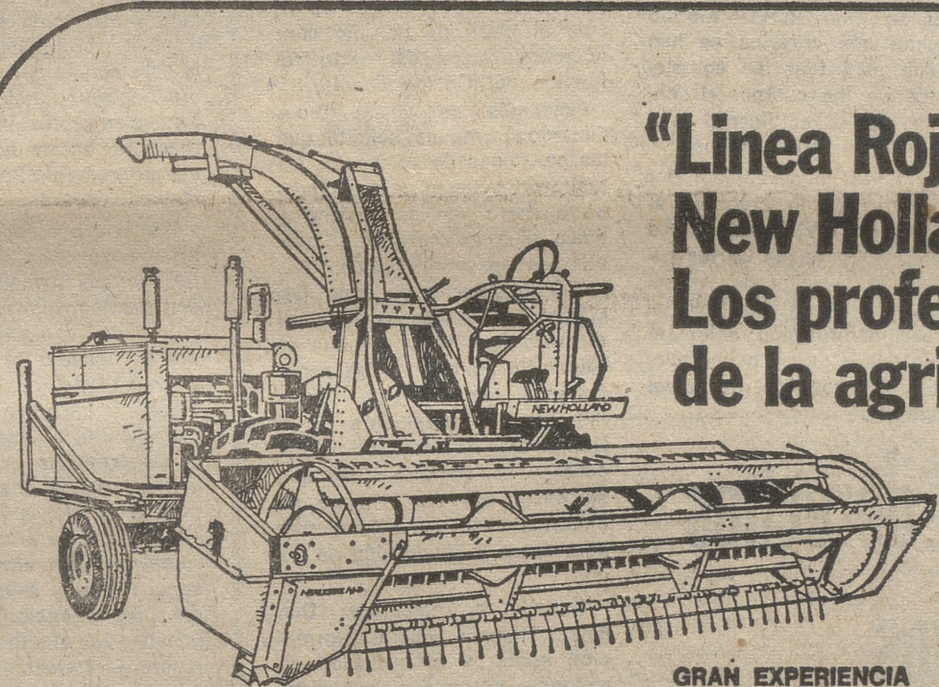
Recogedora Picadora de corte exacto autopropulsada.
