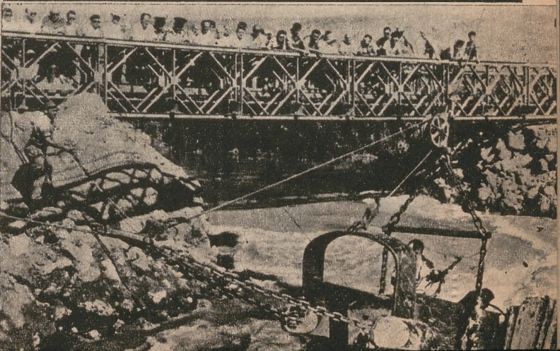
Ingenieros israelíes durante los trabajos de desecación del lago de Hula
