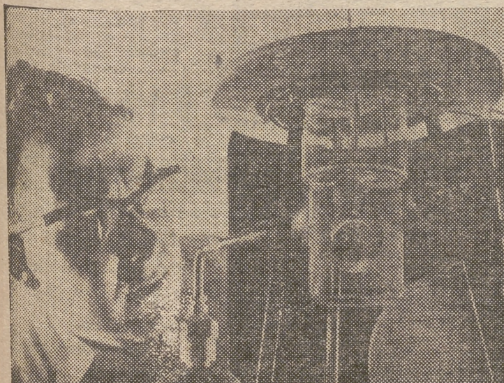
Un científico procede a aplicar un soplete alrededor de un circuito electrónico de los empleados en los nuevos proyectiles dirigidos y aviones supersónicos, para probar si las temperaturas al rojo pueden penetrar en los mencionados circuitos cuando los proyectiles y aviones se hallen a altas estratosféricas. (Foto Cifra.)
