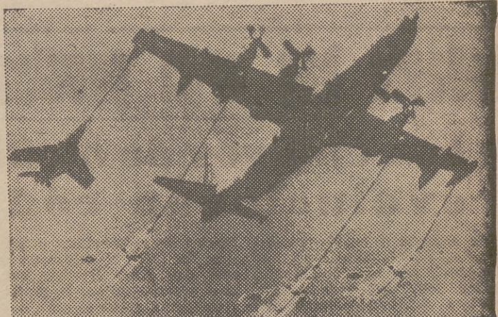
San Diego (California).—Cuatro cazas de propulsión de las Fuerzas Aéreas de la Marina se repostan de gasolina desde una «Convair R3Y-2 Tradewind», en la primera operación múltiple de suministro de esencia en pleno vuelo. El «Tradewind», de 80 toneladas, transporta en sus depósitos gasolina bastante para suministrar a ocho aparatos de combate. Se tardó menos de cinco minutos en la operación. El «Tradewind» pertenece a una escuadra de once aparatos construida en San Diego, con destino a la Marina. — (Foto Cifra Gráfica)
