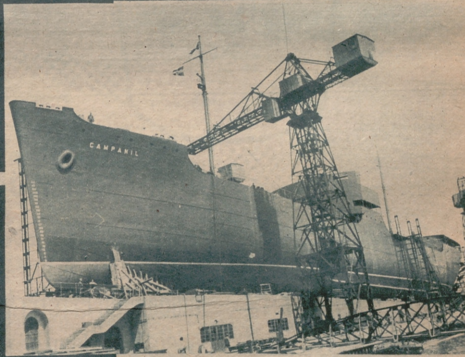
El buque petrolero «Campanil», construido en nuestros astilleros y que mañana, domingo, será botado al agua
